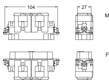
lato contatti (vista anteriore)
