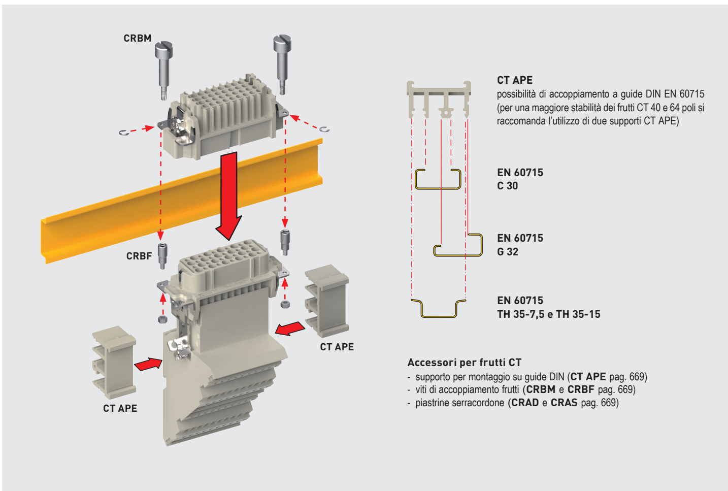
Figura 5 (montaggio su guida DIN)
