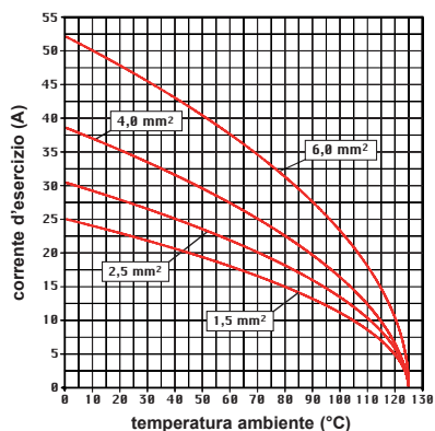
Frutti connettori CP 12 poli Diagramma di derating – massima portata di corrente
