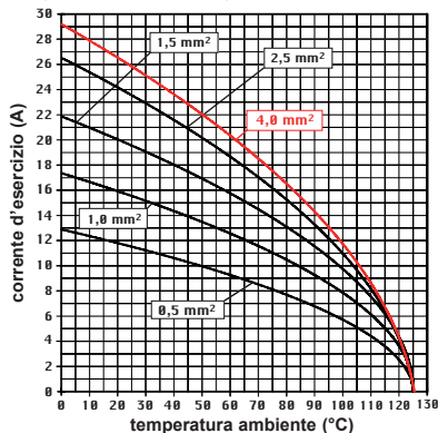
Frutti connettori CMCE 20 poli Diagramma di derating – massima portata di corrente
